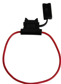
Держатель флажкового предохранителя влагостойкий ABRO® Masters
